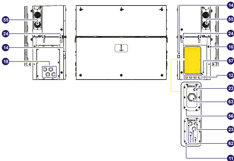
Modulo di potenza PVS-100/120-TL - B2
