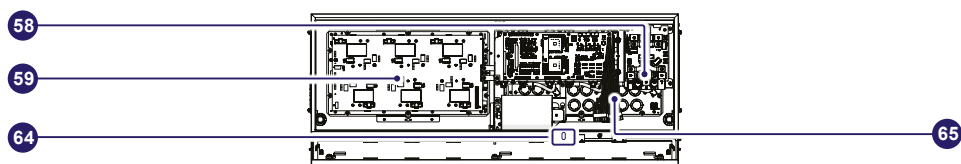
Wiring box con copertura interna PVS-100/120-TL - B2
