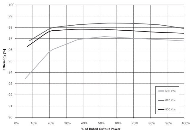
Curva di efficienza TRIO-20.0-TL-OUTD
