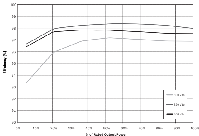
Curva di efficienza TRIO-27.6-TL-OUTD
