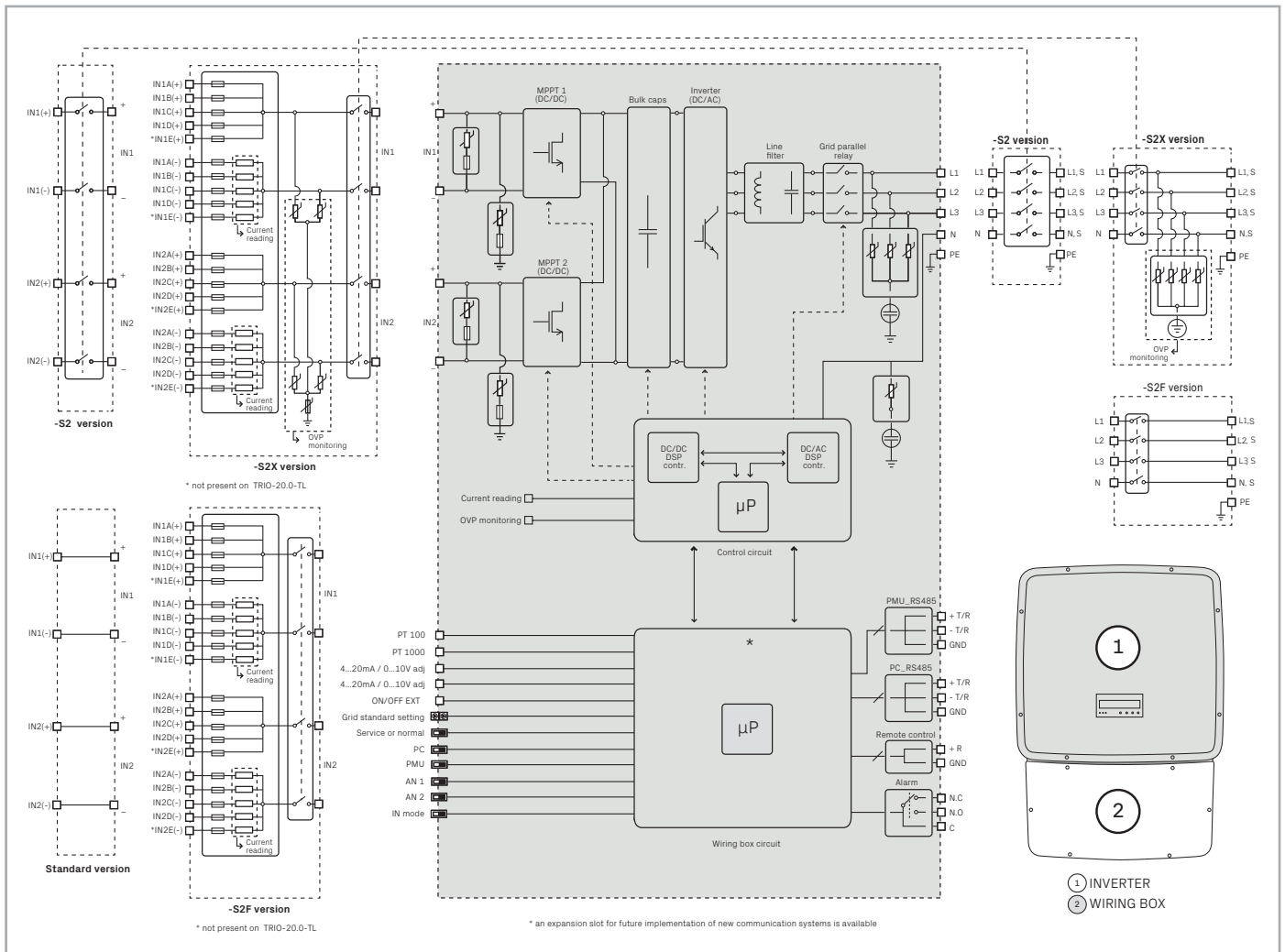
TRIO-20.0/27.6-TL-OUTD diagramma a blocchi
