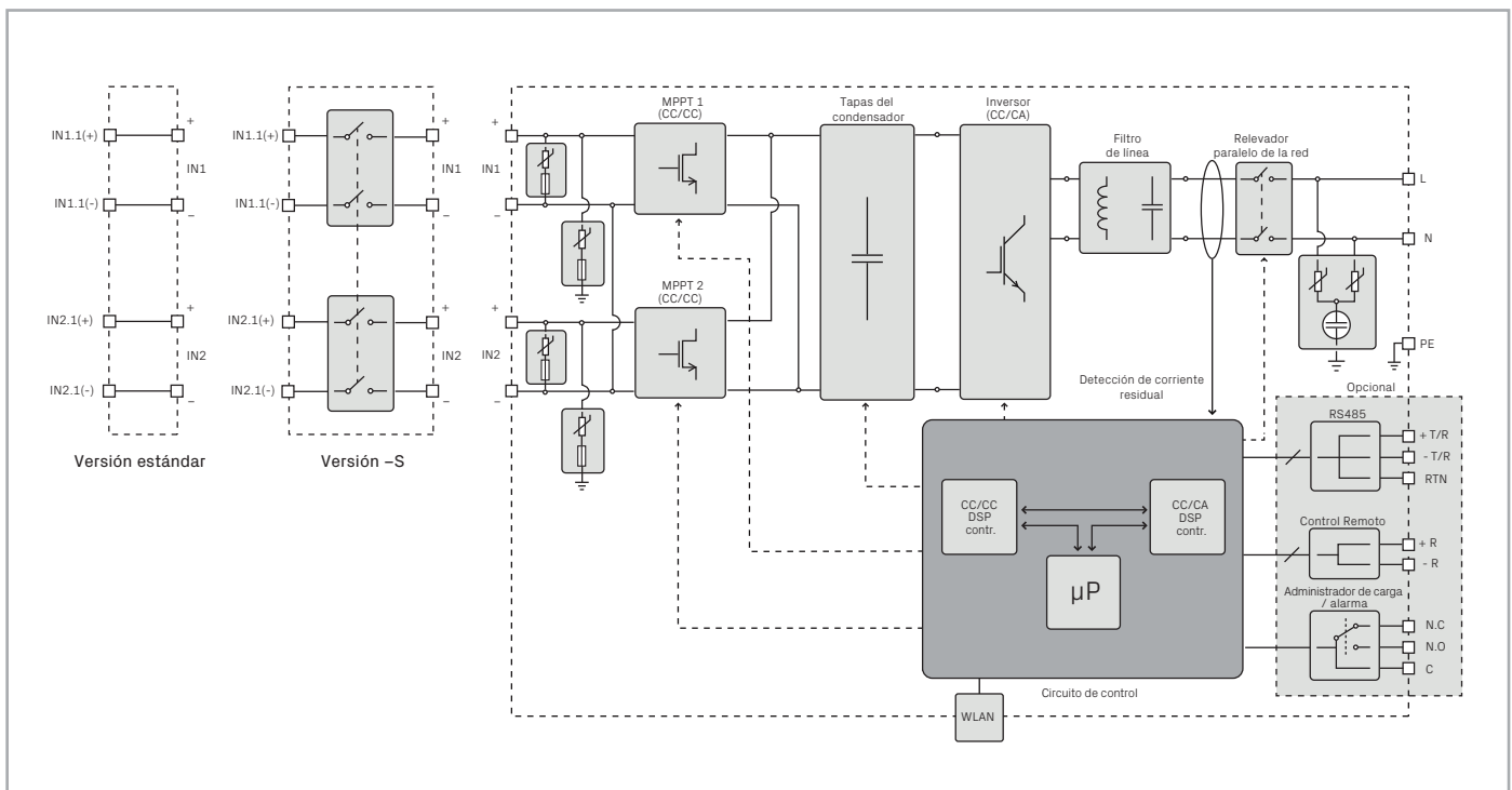
Diagrama de bloques del inversor de cadena UNO-DM-3.3/4.0/4.6/5.0-TL-PLUS-Q
