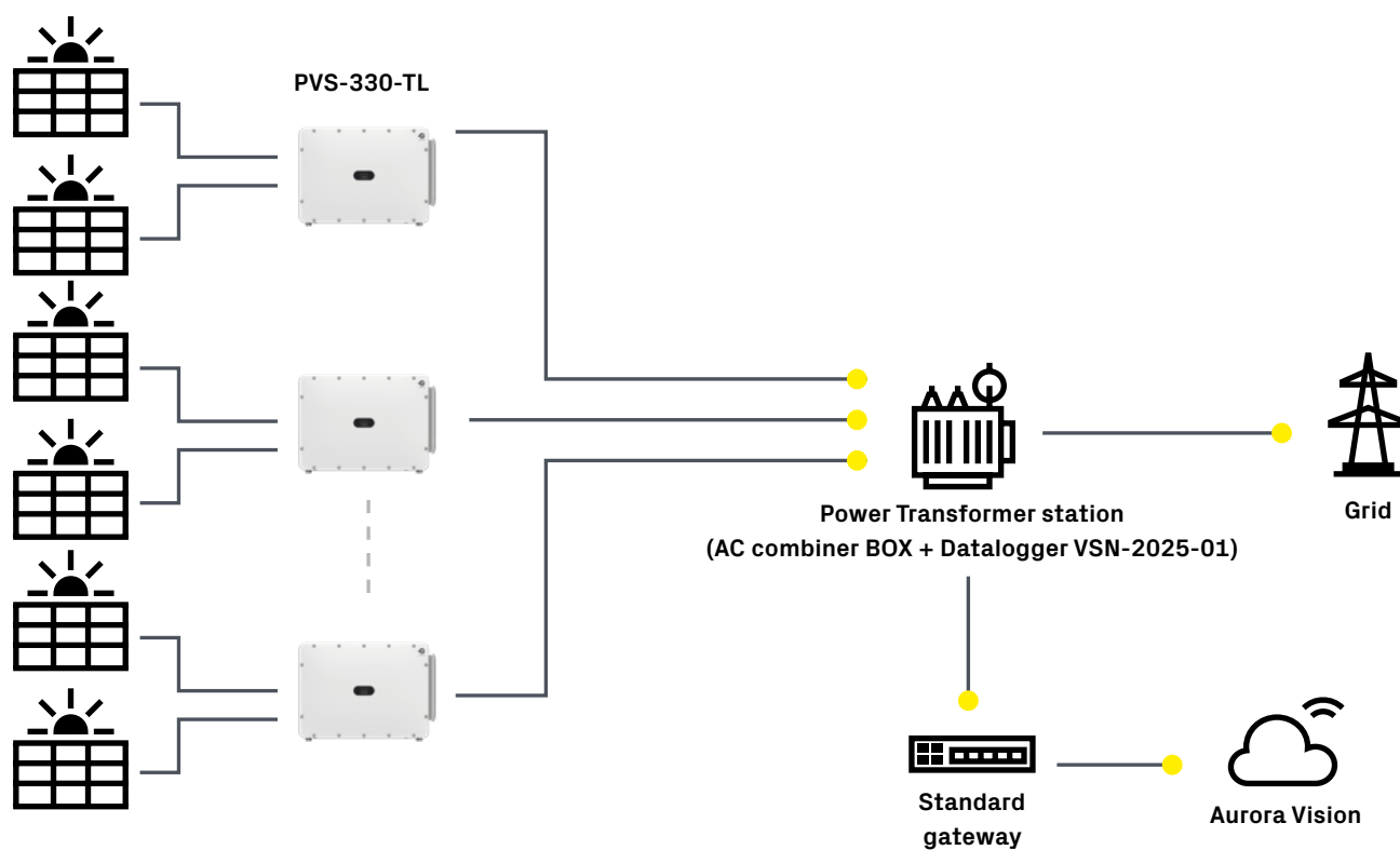
FIMER PVS-330.0 diagramma a blocchi
